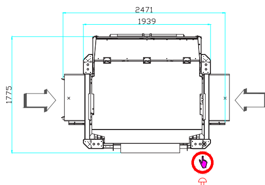
Hauteur de la machine 1840 mm
